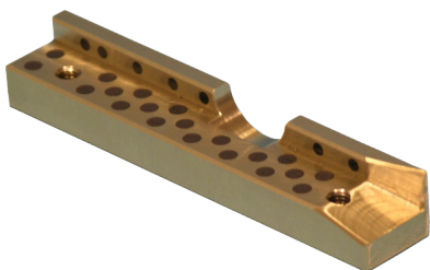
Sonder-Winkelleiste
